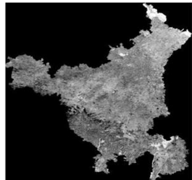
Fig. 3.9 MODIS data NDVI Nov. 2022
