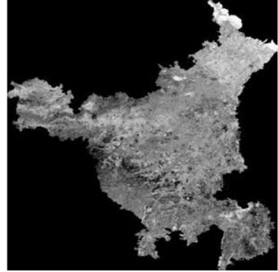
Fig. 3.3 MODIS data NDVI Nov. 2016
