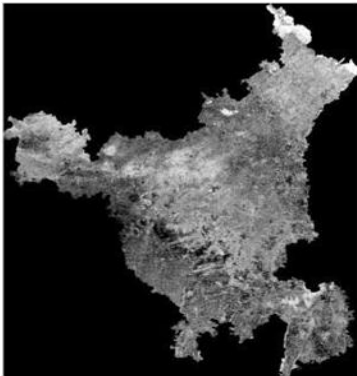
Fig 3.7 MODIS data NDVI Nov. 2020
